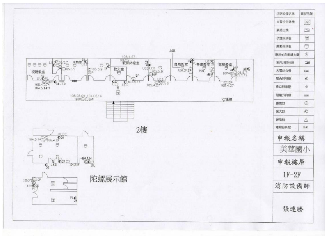
圖 5-2 校園消防安全設施配置圖
